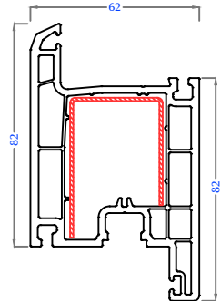
Door Sash - Inward Open PC62-US-04
